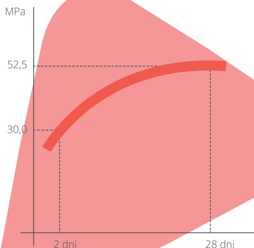
Krzywa Rozwoju Wytrzymałości na Ściskanie · Wartości Minimalne
